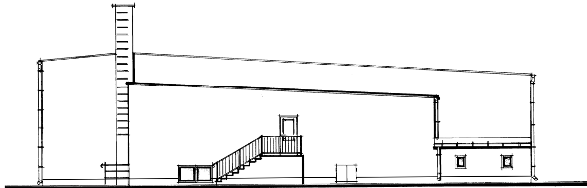
elewacja południowo - wschodnia s. 1:100
